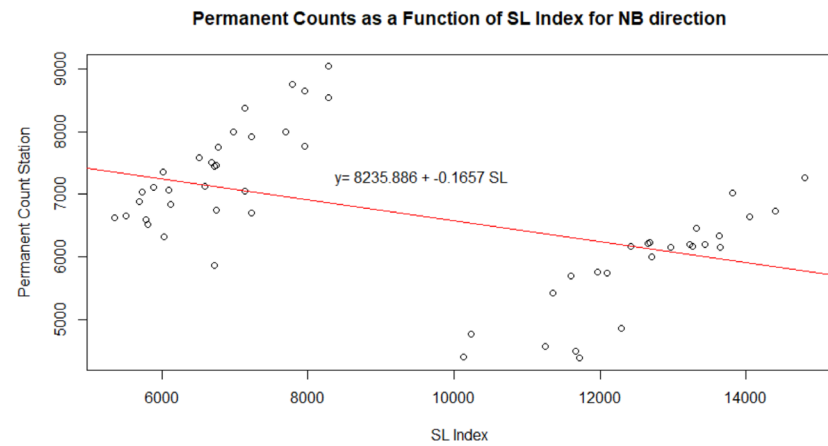
(d) For NB Direction
