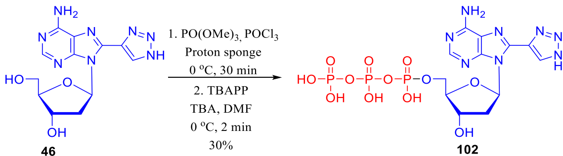
Scheme 28. Synthesis of TrzdATP
